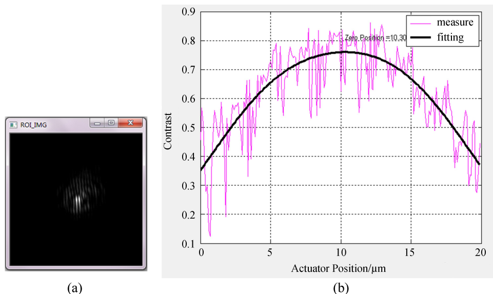
图8 经相机旋转后。(a) 实验采集条纹图;(b) 沿条纹法向行采样得到的对比度变化曲线
